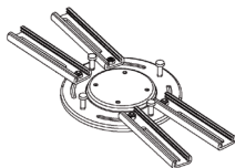
1x projektor fästplatta E
