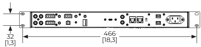
Rückansicht
