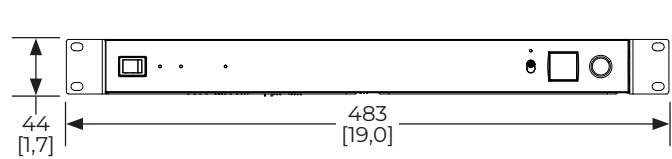
Vorderansicht
