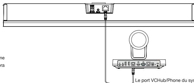
Le port VCHub/Phone du système de visioconférence ou le port Microphone de la caméra de la série UVC.
