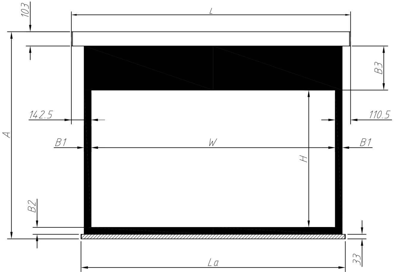
Frontansicht
