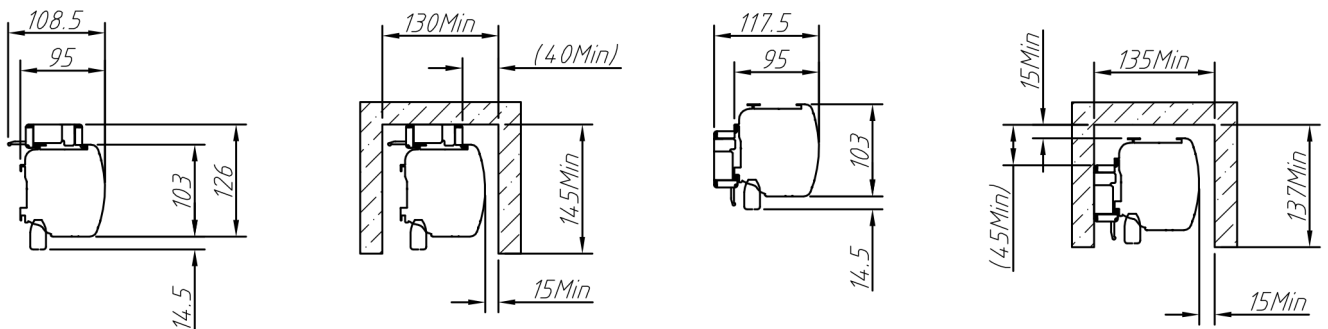
Deckenmontage
