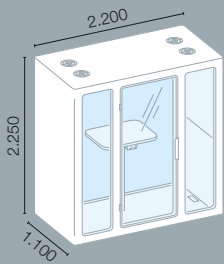
Duo Pod (mit Stehtisch)
