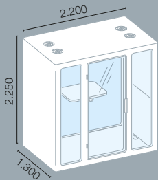
Meeting S (mit Stehtisch)
