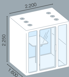
Meeting M (mit Stehtisch)
