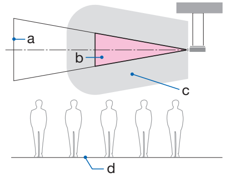
a: Projektionsfläche/B: Gefahrenbereich/c: Vorsorgebereich/d: Fußboden
