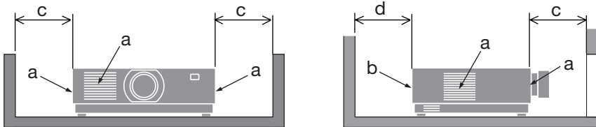
a: Einlassöffnung/b: Auslassöffnung/c: 20 cm oder mehr/ d: 30 cm oder mehr
