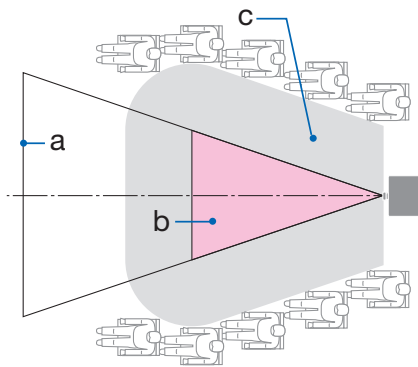
a: Projektionsfläche/B: Gefahrenbereich/c: Vorsorgebereich/d: Fußboden
