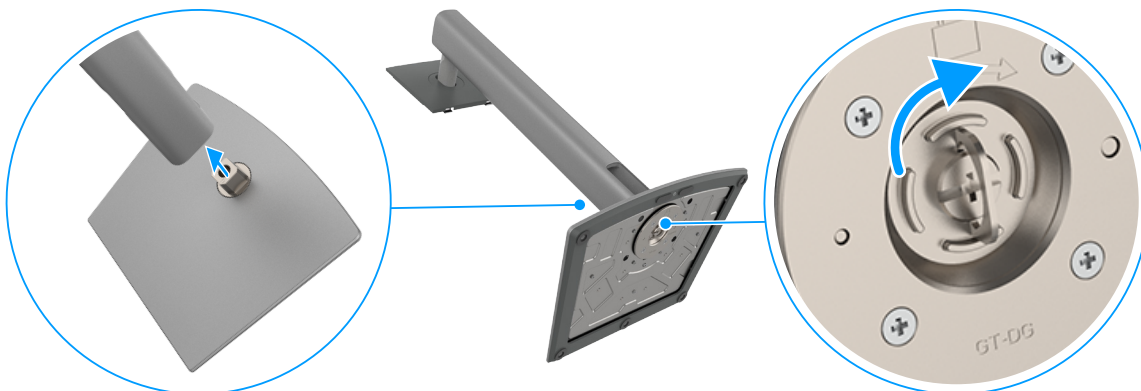
Abbildung 18. Ständer anschließen
