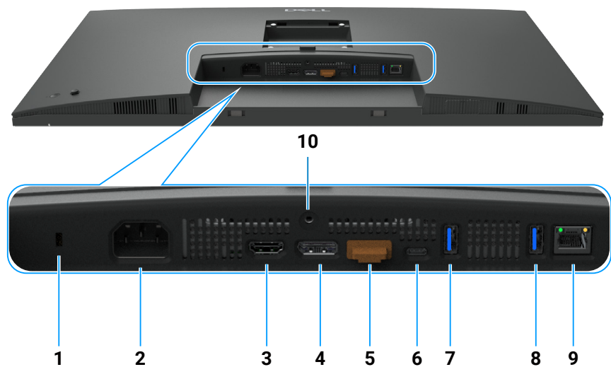
Abbildung 3. Unteransicht des Monitors
