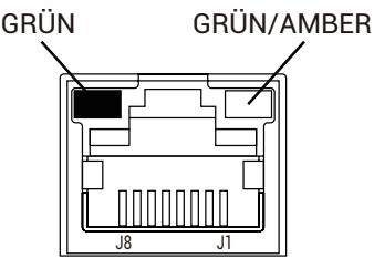
Abbildung 13. RJ45 Port-Konnektor
