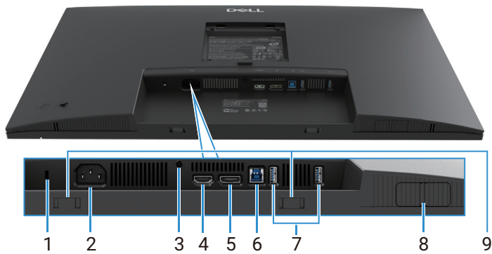
Abbildung 4. Ansicht von unten ohne Monitorstandfuß
