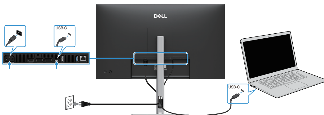
Abbildung 29. USB-C-zu-C-Kabel anschließen
