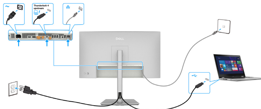
Abbildung 39. Netzwerk-Routing über Thunderbolt 4-Upstream-Anschluss
