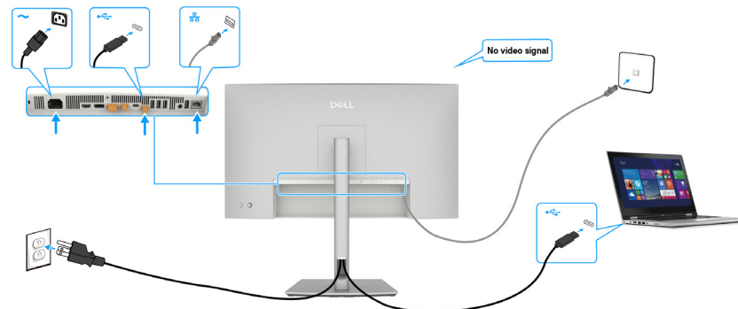
Abbildung 38. Netzwerk-Routing über USB-C-Upstream-Anschluss
